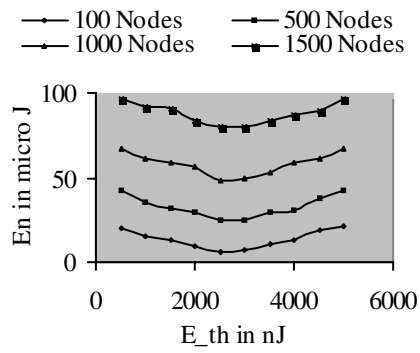
Fig. 2. Poisson Distribution
